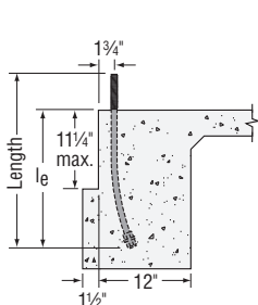
Slab Edge
