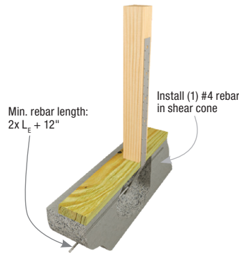
Typical HPAHD22 single pour midwall installation
