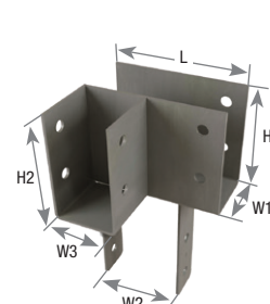
KECCL left shown
